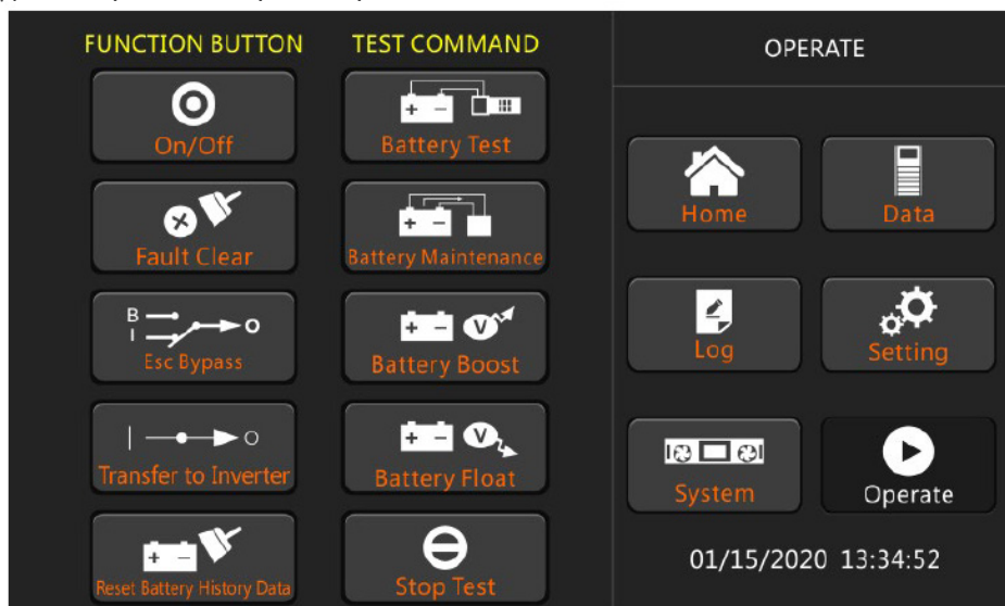
Рис. 6-1 Страница Батарей
