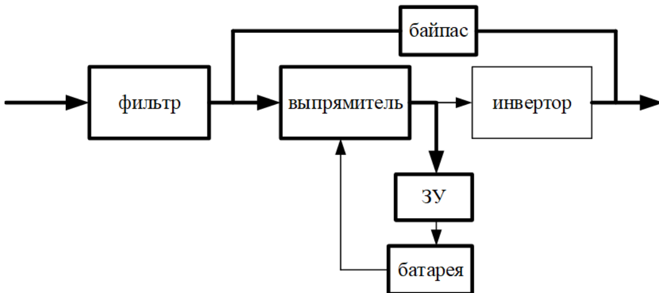
Рис. 3-3 Режим байпаса
