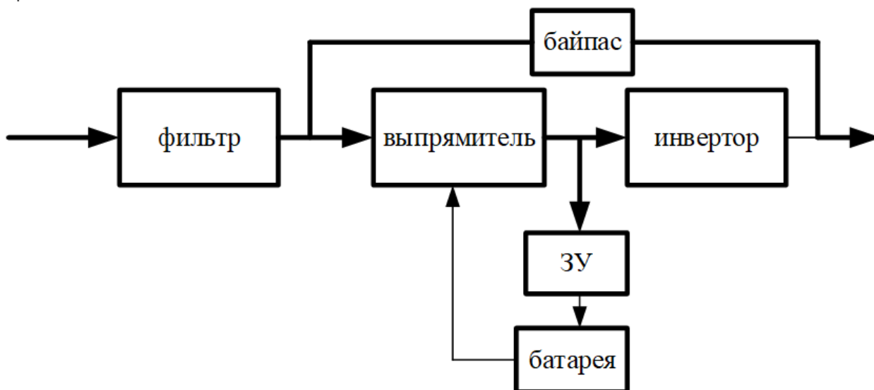
Рис. 3-5 ECO режим
