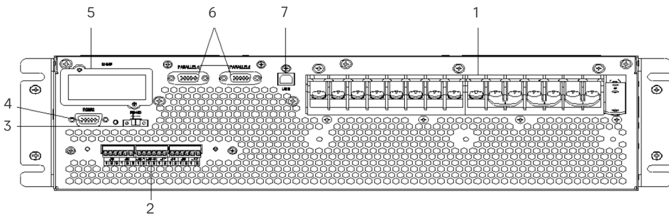
Рис. 1-3 Вид сзади 10-20 кВА
