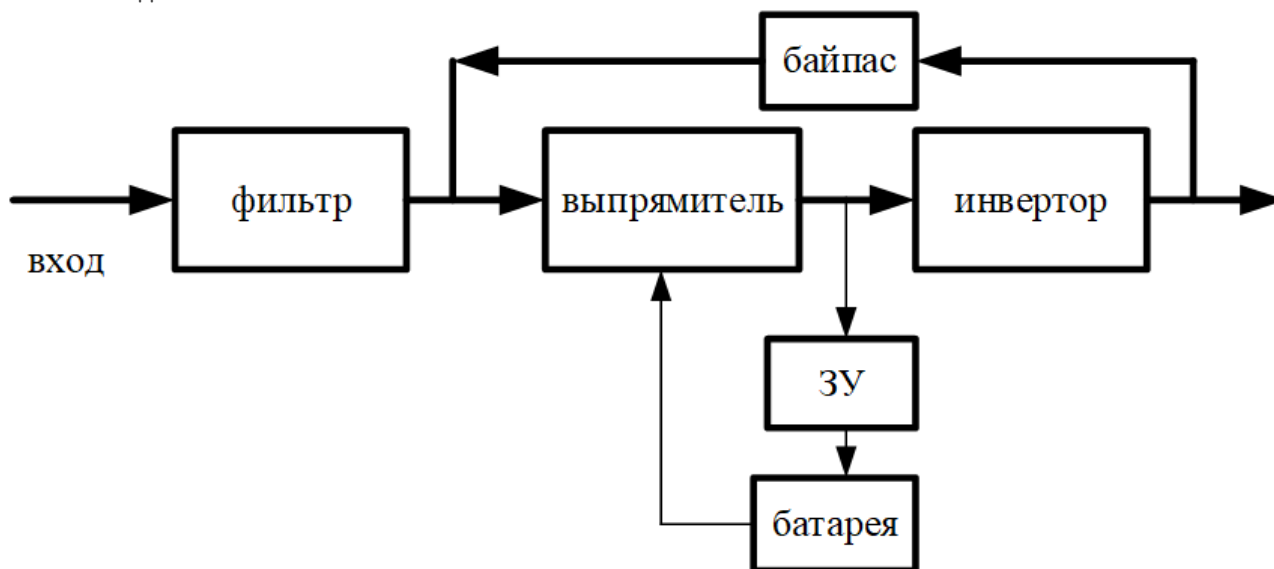
Рис. 3-6 Режим самодиагностики
