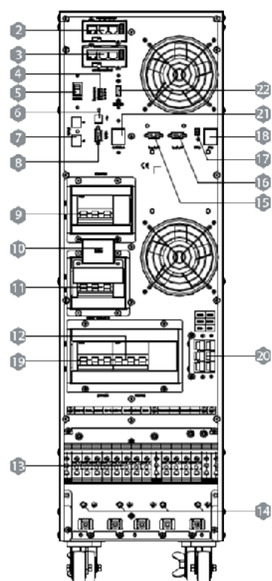
КС3330S (30 кВА) КС3340S (40 кВА)
