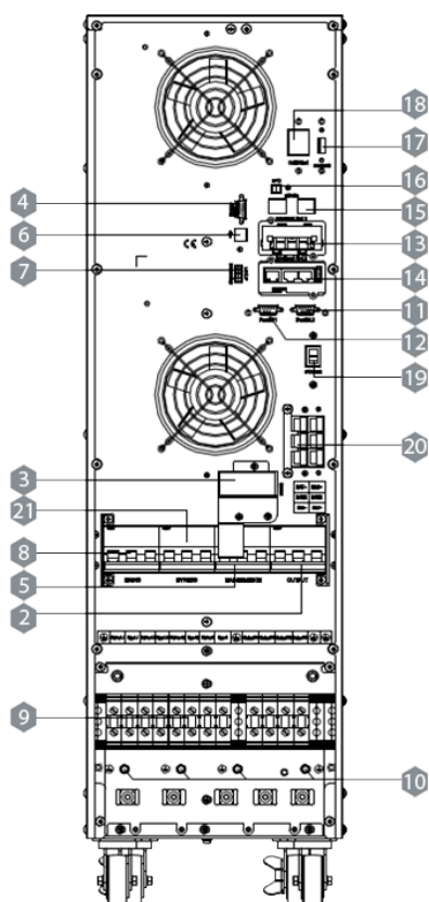
КС3310S (10 кВА) КС3315S (15 кВА) КС3320S (20 кВА)
