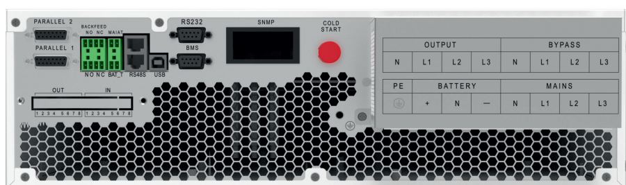
Вид сзади моделей 15-20-30К
